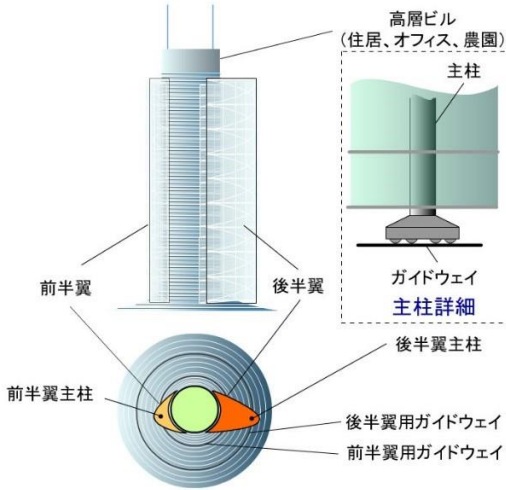
揚力発生装置(高層ビル)の詳細
